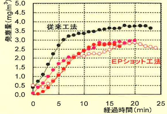
粉じん量測定結果
